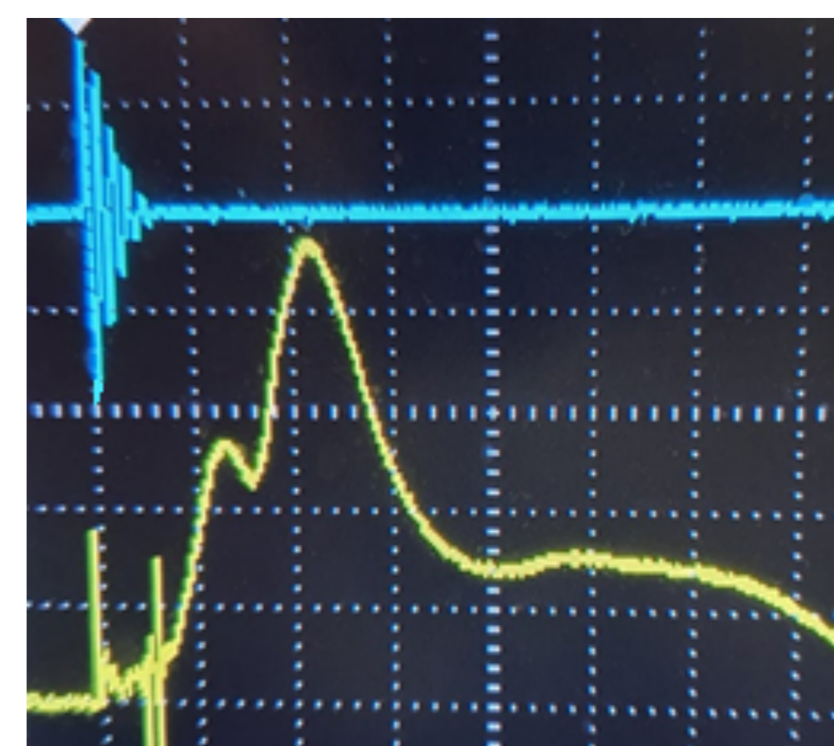
в) верхний луч: ток 32 кА, нижний луч: 20 В/дел
