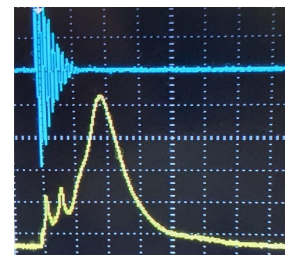
г) верхний луч: ток 42 кА, нижний луч: 50 В/дел
