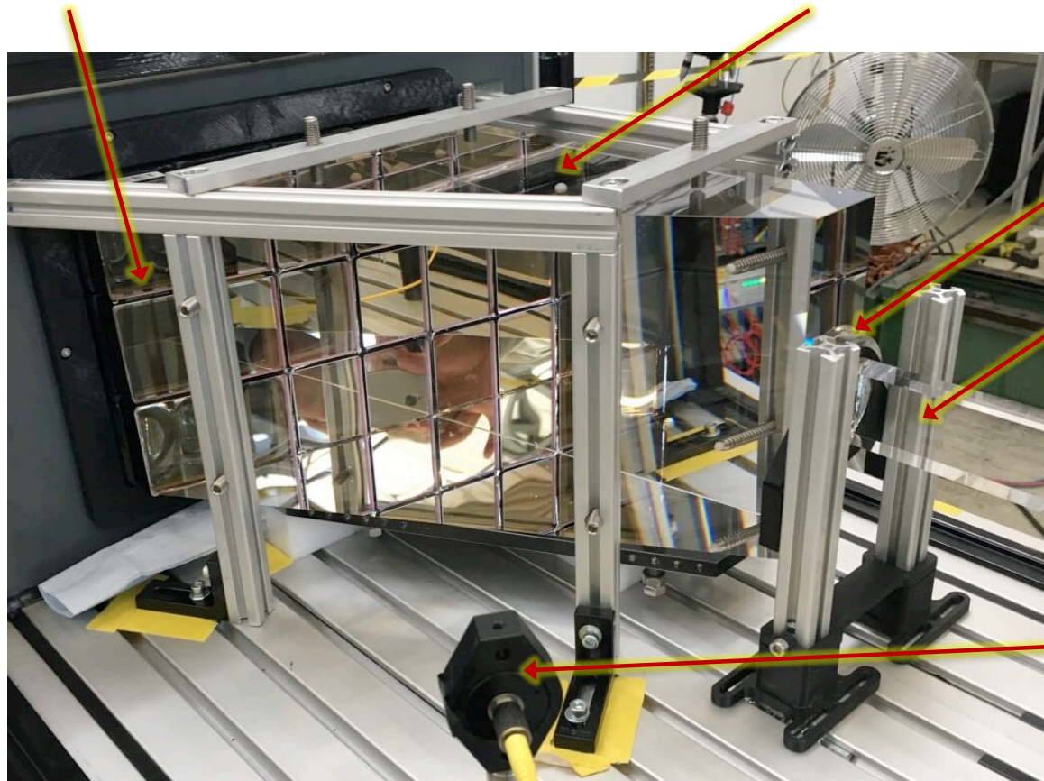
MCP-PMT array
